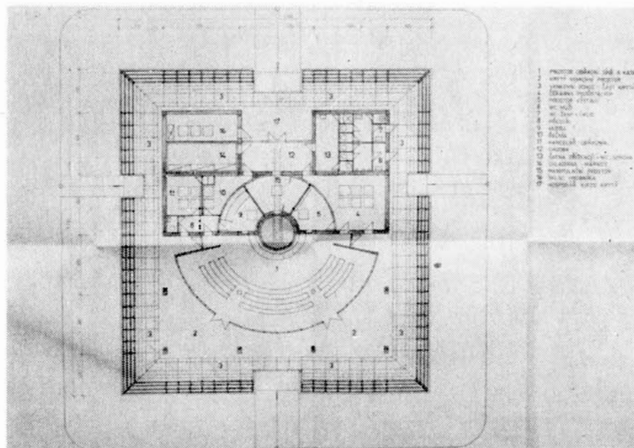
Plán ukazuje půdorys smuteční obřadní síně: vstup, ochoz kolem obřadní místnosti, vlastní obřadní místnost + katafalk, místnost pro výstav, obřadníka, řečníka a hudbu atd.
