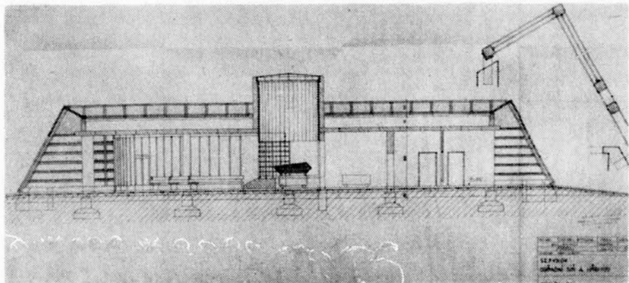
Řez smuteční obřadní síní. Plášť tvoří dřevěná konstrukce, strop a příčky hlavní stavby jsou panelového typu, střední část s katafalkem je nahore kruhově prosklená.
