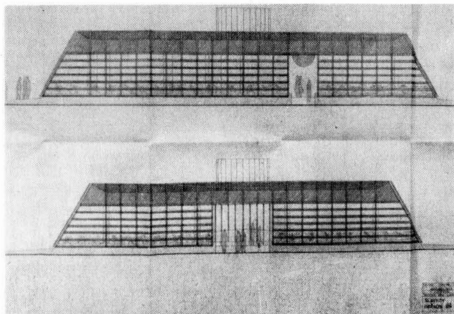
Pohled na průčelí smuteční obřadní síně — východní strana (objekt je opláštěván dřevěnou pergolou, která je v horní části prosklena barevným sklem). Druhý snímek ukazuje hlavní vstup ze západní strany
