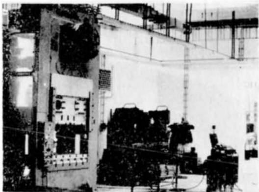
Na obrázku 315tunový tvářecí lis pro výrobu součástí a dílů kotlů i dalších výrobků. Ze záběru je vidět vybavení a světlost haly, v níž je lis umístěn.
